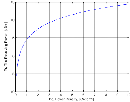
Şekil.2.b f=900MHz
